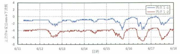
図-18 2020年6月11日～18日における測点1の動き
