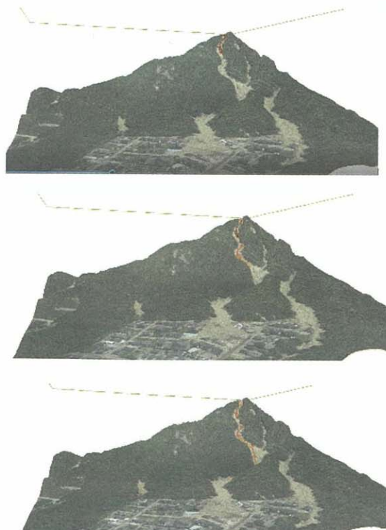
図-9 三次元土石流シミュレーションの結果例 (土石流を赤で表示, 上から下へ流出過程を示す. 写真は国土地理院による)
