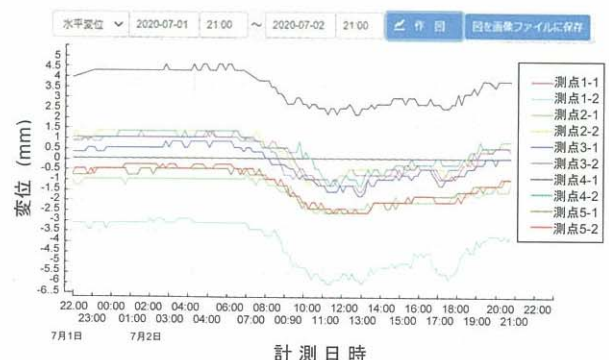
図-16 溪流内地盤変位経時変化図の表示例
