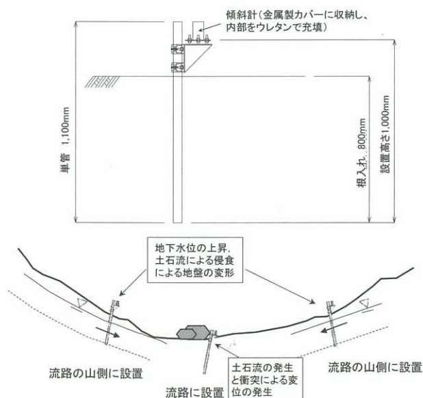
図-3 傾斜計を用いた土石流センサーの構造と溪流における地盤変位の計測
