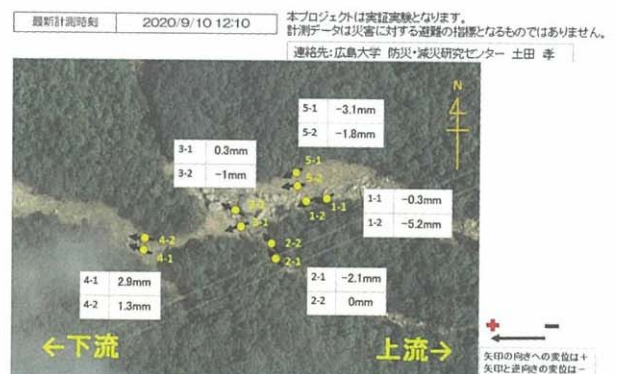
図-15 溪流内の地盤変位の表示例(写真は国土地理院による)
