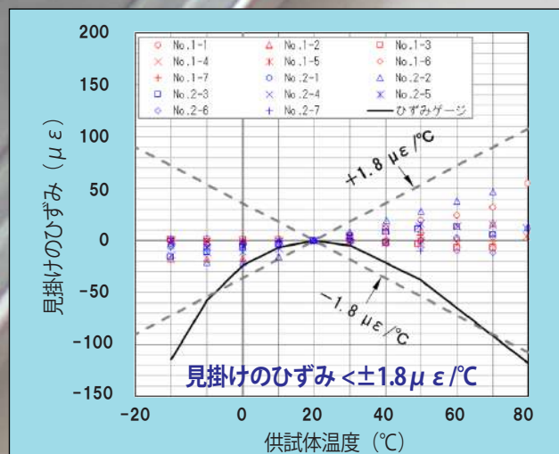
試験体：鋼製板 (線膨張係数) 11.7 \mu\epsilon/^\circ\text{C}
