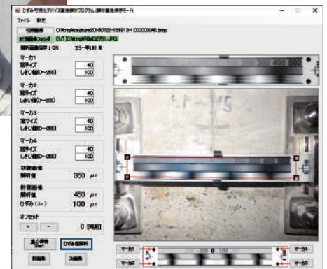
画像解析プログラム
