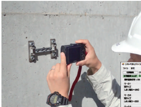
デジタルカメラによる 写真撮影
